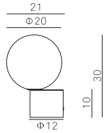
MT10563-1-200ST 燈體尺寸：21×20×30 功 率：G9 1×3.5W 材 質：銅+玻璃 顏 色：銅本色
