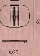
MT21910-1-250A 灯体尺寸: \phi 25 \times 35 cm 功 率: LED 11W 材 质: 金属+玻璃 颜 色: 烤漆半光枪黑+烟灰色
