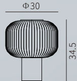
MT95191-1-300 灯体尺寸：Φ30×34.5CM 功 率：E27×1 材 质：洞石+玻璃 颜 色：奶白+米黄
