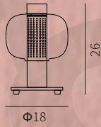
MT21910-1-180A 灯体尺寸: \phi 18 \times 26 功 率: LED 8W 材 质: 金属+玻璃 颜 色: 烤漆半光枪黑+烟灰色
