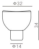
MT10872-1-320 燈體尺寸：Φ32×34 功 率：LED 7.5W 材 質：玻璃+金屬 顏 色：幹邑色
