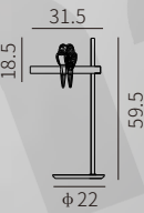
MT80508-1-300 灯体尺寸: 31.5×59.5cm 功 率: LED 17W 材 质: 铝+琉璃 颜 色: 哑光砂镍
