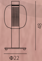
MT21910-1-220B 灯体尺寸: \phi 22 \times 48 cm 功 率: LED 15W 材 质: 金属+玻璃 颜 色: 烤漆半光枪黑+烟灰色
