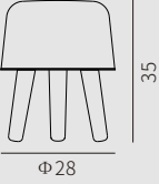
MT21951-1-280 灯体尺寸: \Phi 28 \times 35\text{cm} 功 率: G9 \times 1 (可调光) 材 质: 木头+玻璃+亚克力 颜 色: 原木色+奶
