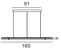
MD80599-1L-1615 灯体尺寸: 160×180cm 功 率: LED 31W 材 质: 铝+K9水晶 颜 色: 哑光砂镍
