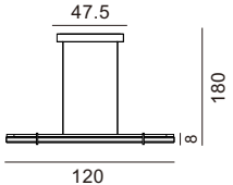
MD80599-1L-1200 灯体尺寸: 120×180cm 功 率: LED 24W 材 质: 铝+K9水晶 颜 色: 哑光砂镍
