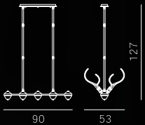
MD60186-10L-900S 燈體尺寸：90×127 功 率：E27 10×4W 材 質：銅+大理石 顏 色：電鍍半光拉絲青銅
