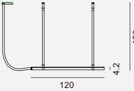
MD54108-1A-1200 灯体尺寸: 120x4.2x150CM 功 率: LED 27W 材 质: 铝+奢石板 颜 色: 哑黑+石材: 贝克斯加
