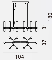
MD80556-20L-1040 灯体尺寸:104×37×180 功 率:G9×20 材 质:西班牙云石+铁 颜 色:枪黑(烤漆)
