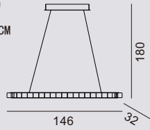
MD80610-1L-1460 灯体尺寸: 146×32×180CM 功 率: LED 72W 材 质: 铝+水晶 颜 色: 哑白
