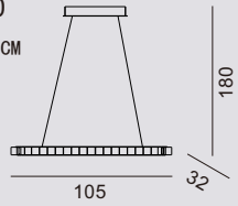
MD80610-1L-1050 灯体尺寸: 105×32×180CM 功 率: LED 52W 材 质: 铝+水晶 颜 色: 哑白
