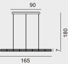
MD80600-1L-1600 灯体尺寸：165×180cm 功 率：LED 50W 材 质：K9水晶 颜 色：氧化亮银
