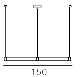
MD23031-1L-1500 灯体尺寸: 150×180cm 功 率: LED 40W 材 质: 铝+西班牙云石 颜 色: 哑光砂镍
