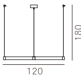
MD23031-1L-1200 灯体尺寸: 120×180cm 功 率: LED 33W 材 质: 铝+西班牙云石 颜 色: 哑光砂镍
