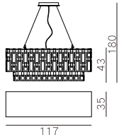
MD80200-6L-1170 燈體尺寸：117×35×180 功 率：E14 6×40W 材 質：金屬+手工玻璃 顏 色：馬斯登專用金
