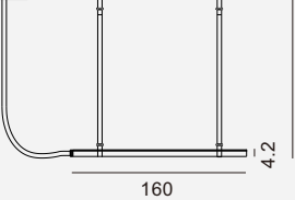
MD54108-1B-1600 灯体尺寸: 160x4.2x150CM 功 率: LED 37W 材 质: 铝+奢石板 颜 色: 哑黑+石材: 流金水月
