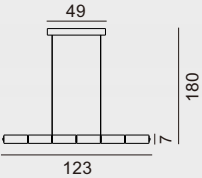
MD80600-1L-1200 灯体尺寸：123×180cm 功 率：LED 37W 材 质：K9水晶 颜 色：氧化亮银
