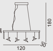
MD21880-1L-1200 灯体尺寸: 120×30×180cm 功 率: LED 63W 材 质: 金属+不锈钢+水晶+玻璃 颜 色: 镀铬+清光
