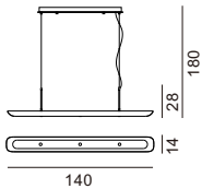
MD21850-1L-1400 灯体尺寸: 140×14×180 功 率: LED 材 质: 铜+云石 颜 色: 双面拉丝封半光油
