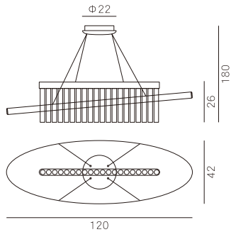
MD23016-2L-1200A 灯体尺寸: 120×42×180cm 功 率: LED 85W 材 质: 铁+铝+亚克力 颜 色: 电镀枪黑封亮油
