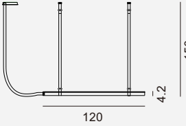
MD54108-1B-1200 灯体尺寸: 120x4.2x150CM 功 率: LED 27W 材 质: 铝+奢石板 颜 色: 哑黑+石材: 流金水月
