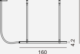
MD54108-1A-1600 灯体尺寸: 160x4.2x150CM 功 率: LED 37W 材 质: 铝+奢石板 颜 色: 哑黑+石材: 贝克斯加
